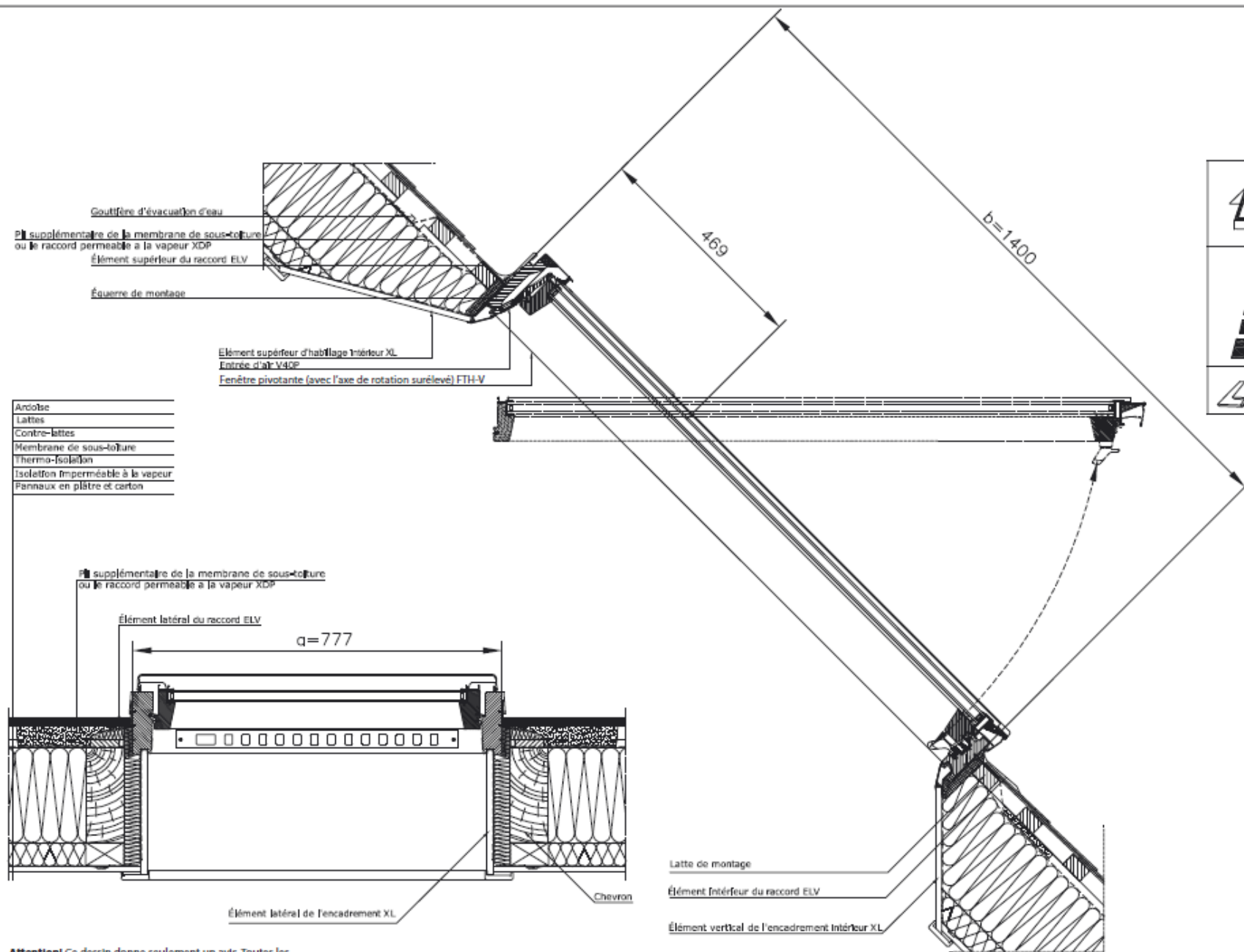
COUPE VERTICALE ET HORIZONTALE: FENÊTRES PIVOTANTE FTH-V (AVEC L'AXE DE ROTATION SURÉLEVÉ) AVEC RACCORD D'ÉTANCHÉITÉ ELV POUR LES COUVERTURES PLATES
