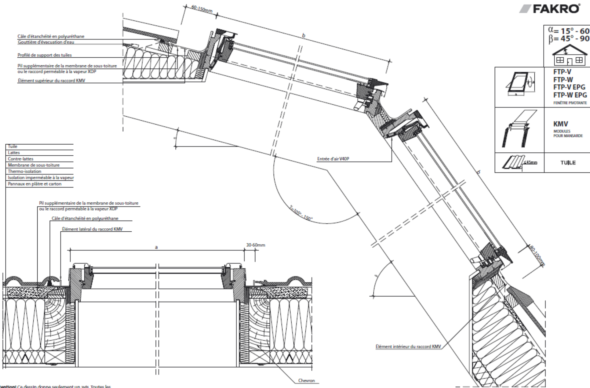
COUPE VERTICAL ET HORIZONTALE: FENÊTRE PIVOTANTE FTP-V/ EPG, FTP-W/ EPG AVEC MODULES POUR MANSARDE KMV
