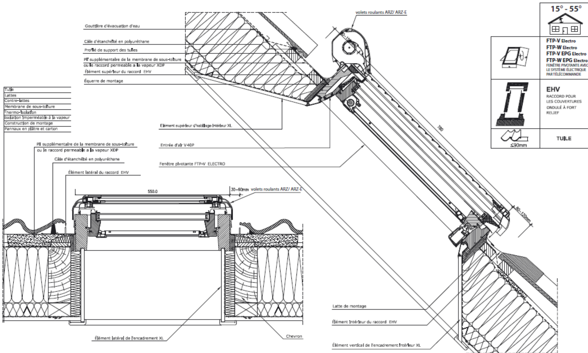
COUPE VERTICAL ET HORIZONTALE: FENÊTRE PIVOTANTE FTP-V/ EPG Electro, FTP-W/ EPG Electro AVEC RACCORD D'ÉTANCHÉITÉ EHV POUR LES COUVERTURES À FORT RELIEF
