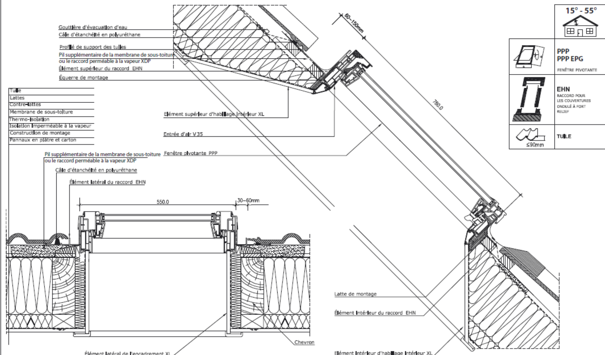
COUPE VERTICAL ET HORIZONTALE: FENÊTRE BASCULANTE-PIVOTANTE PPP/EPG preSelect AVEC RACCORD D'ÉTANCHÉITÉ EHN POUR LES COUVERTURES À FORT RELIEF
