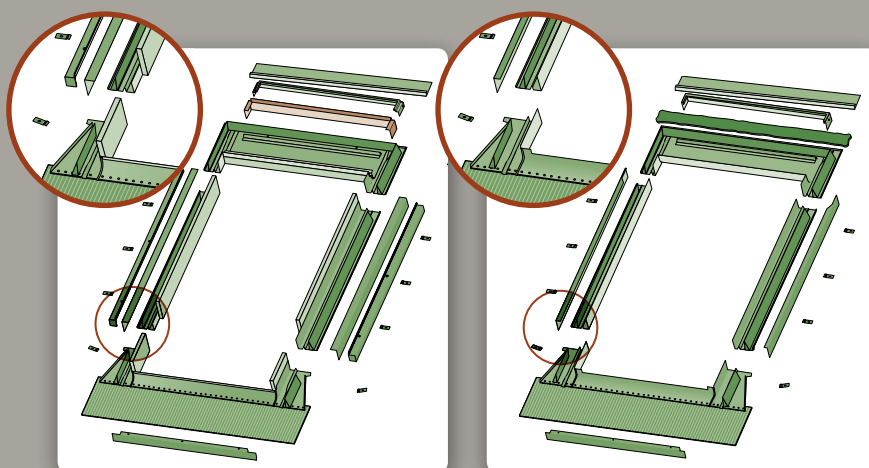
Le raccord d'étanchéité EHU-AT Thermo
